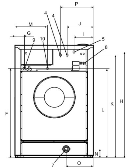
Hátulnézet
