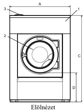
Előlnézet
