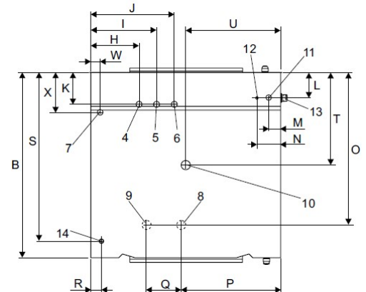
Felülnézet
