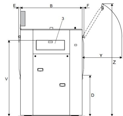
Bal oldalnézet
