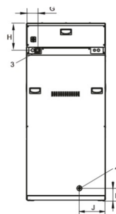
Hátulnézet
