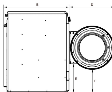
Bal oldalnézet
