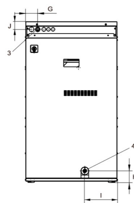
Hátnézet
